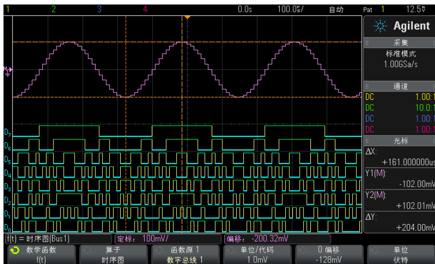
图 18 逻辑图总线时序示例
