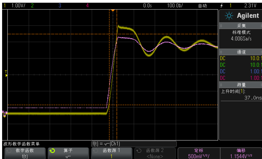
图 10 \sqrt{\quad} (平方根) 的示例
