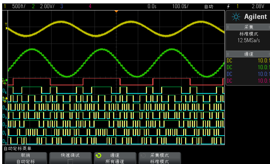
图 20 例如：数字通道的自动定标（仅限于 MSO 型号）
