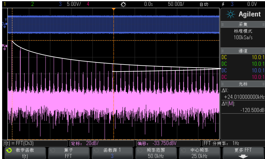
图 9 混叠
