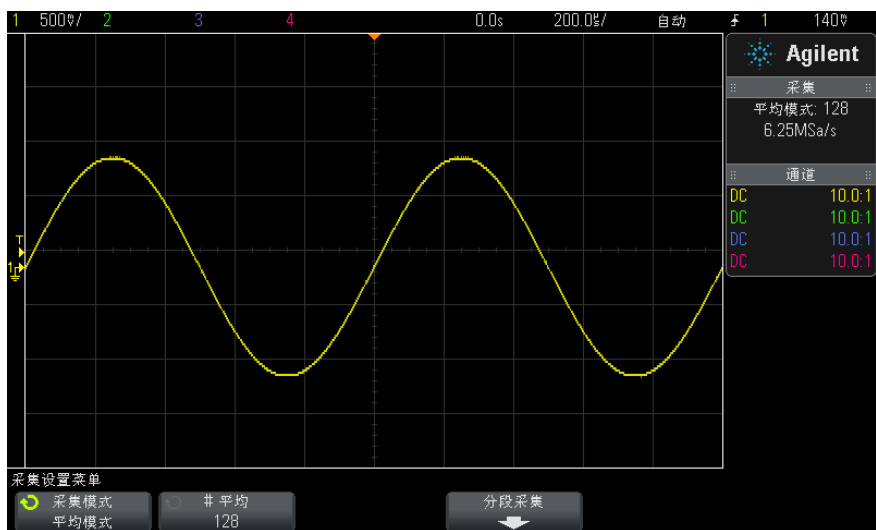
图 39 用于降低随机噪声的平均数 128
