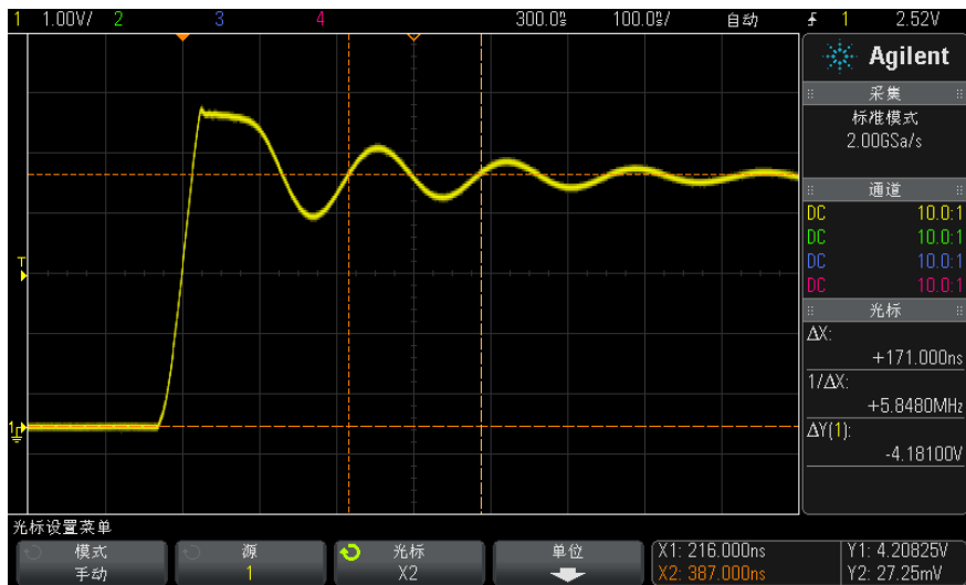
图 41 光标测量脉冲振铃频率
