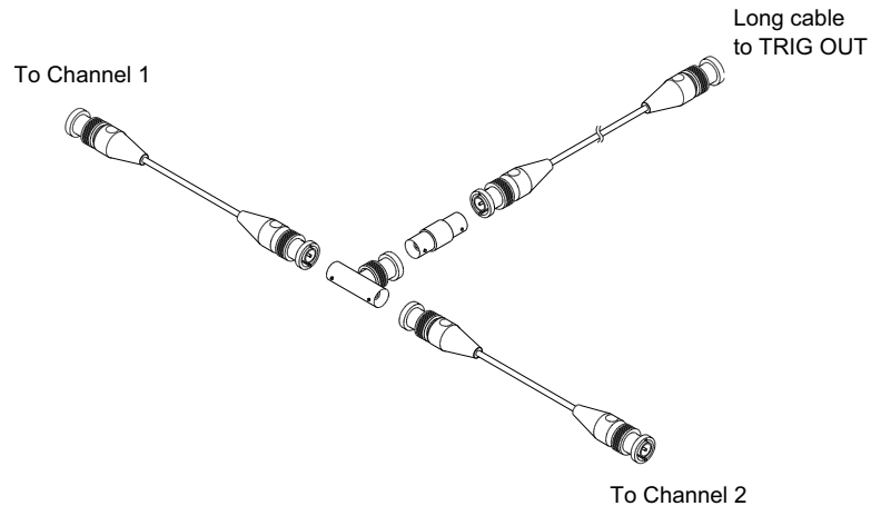
图 48 用于 2 通道示波器的用户校准电缆
